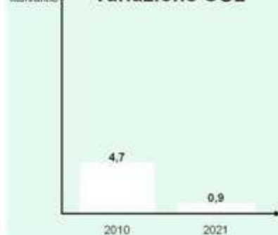
Variatione CO2
