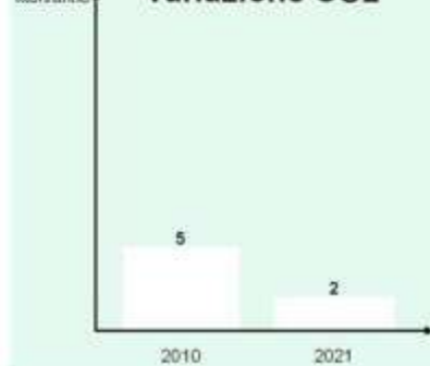
Variation CO2
