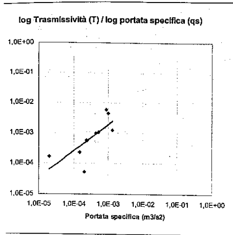
Figura 13 - Diagramma logaritmico per la determinazione della relazione tra trasmissività e portata specifica.
