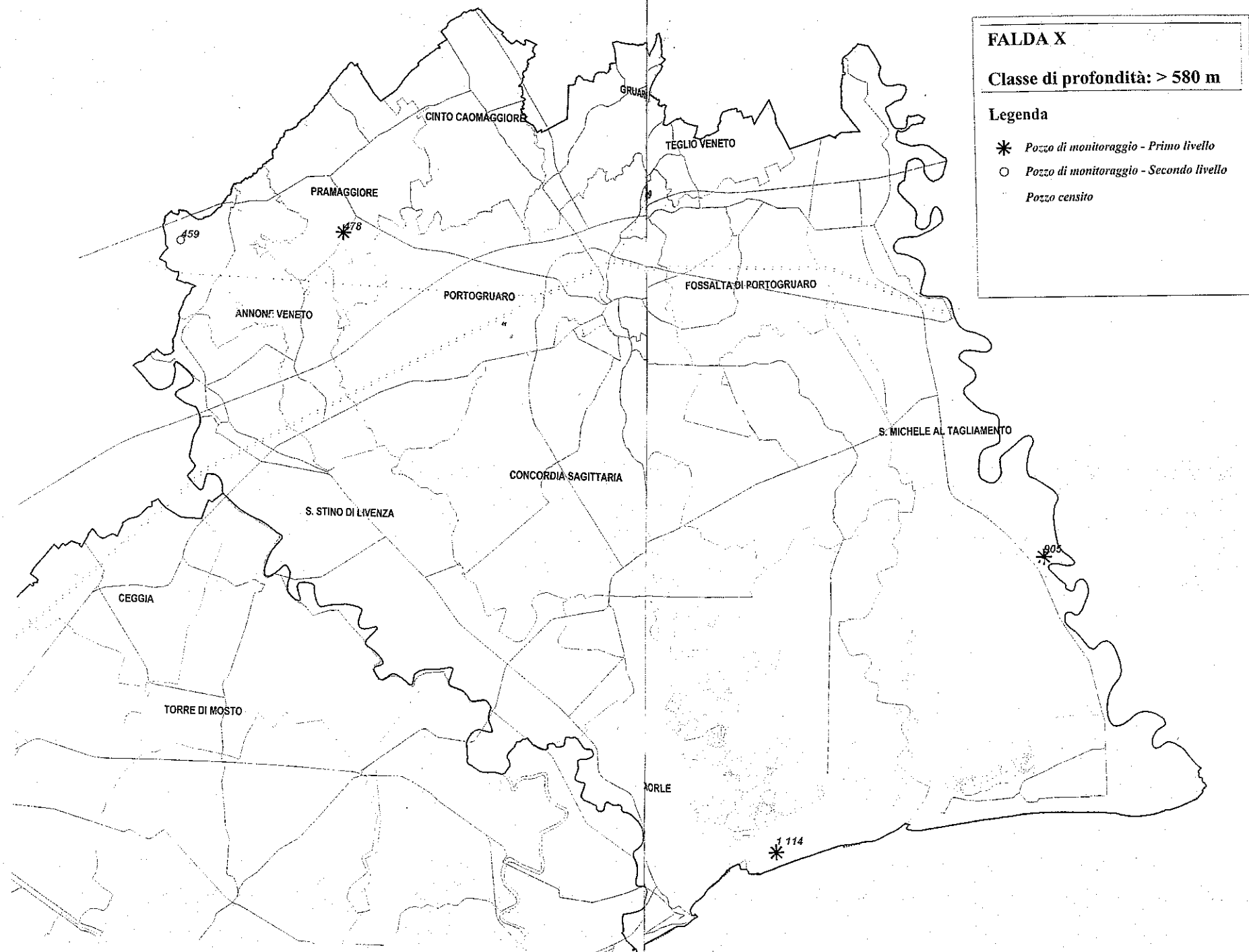
Figura 42 - Falda X - Classe di profondità: > 580 m. Pozzi censiti e rete di monitoraggio.
