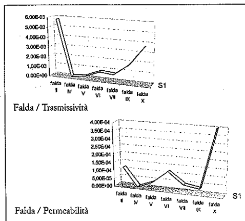
Figura 12 - Valore medio misurato di trasmissività e permeabilità per ciascuna falda.
