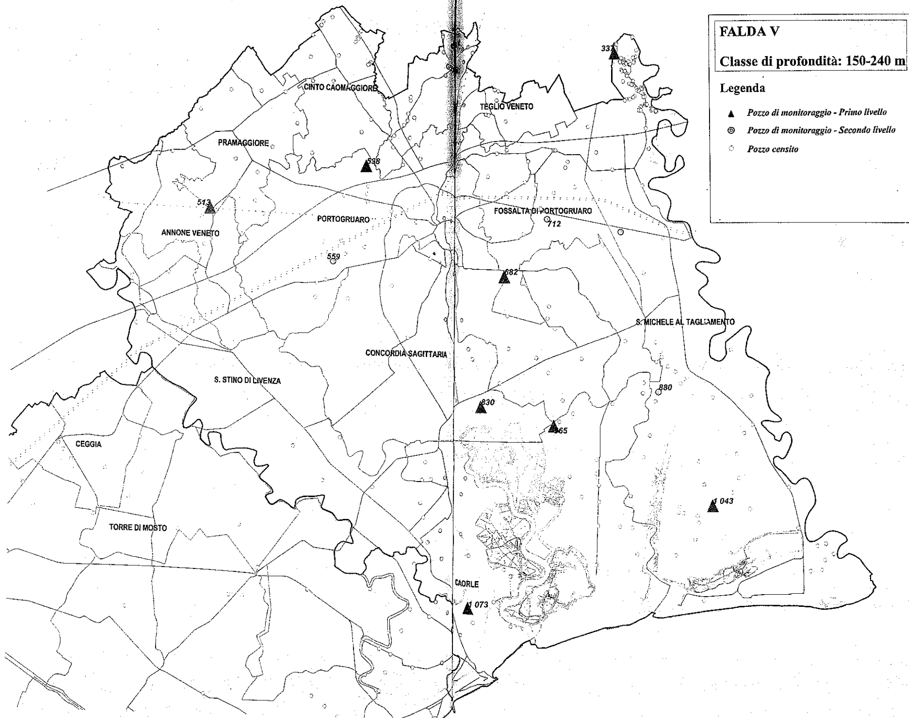
Figura 37 - Falda V - Classe di profondità: 150-240 m. Pozzi censiti e rete di monitoraggio.
