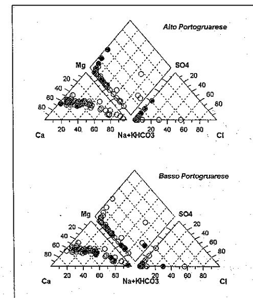
Figura 19 - Diagrammi di Piper (da Zangheri, 2000)
