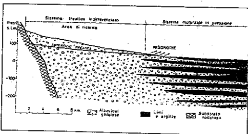
Figura 2 - Modello idrogeologico della Pianura Veneto-Friulana. La figura rappresenta uno spaccato (sezione) con direzione Nord-Sud.
