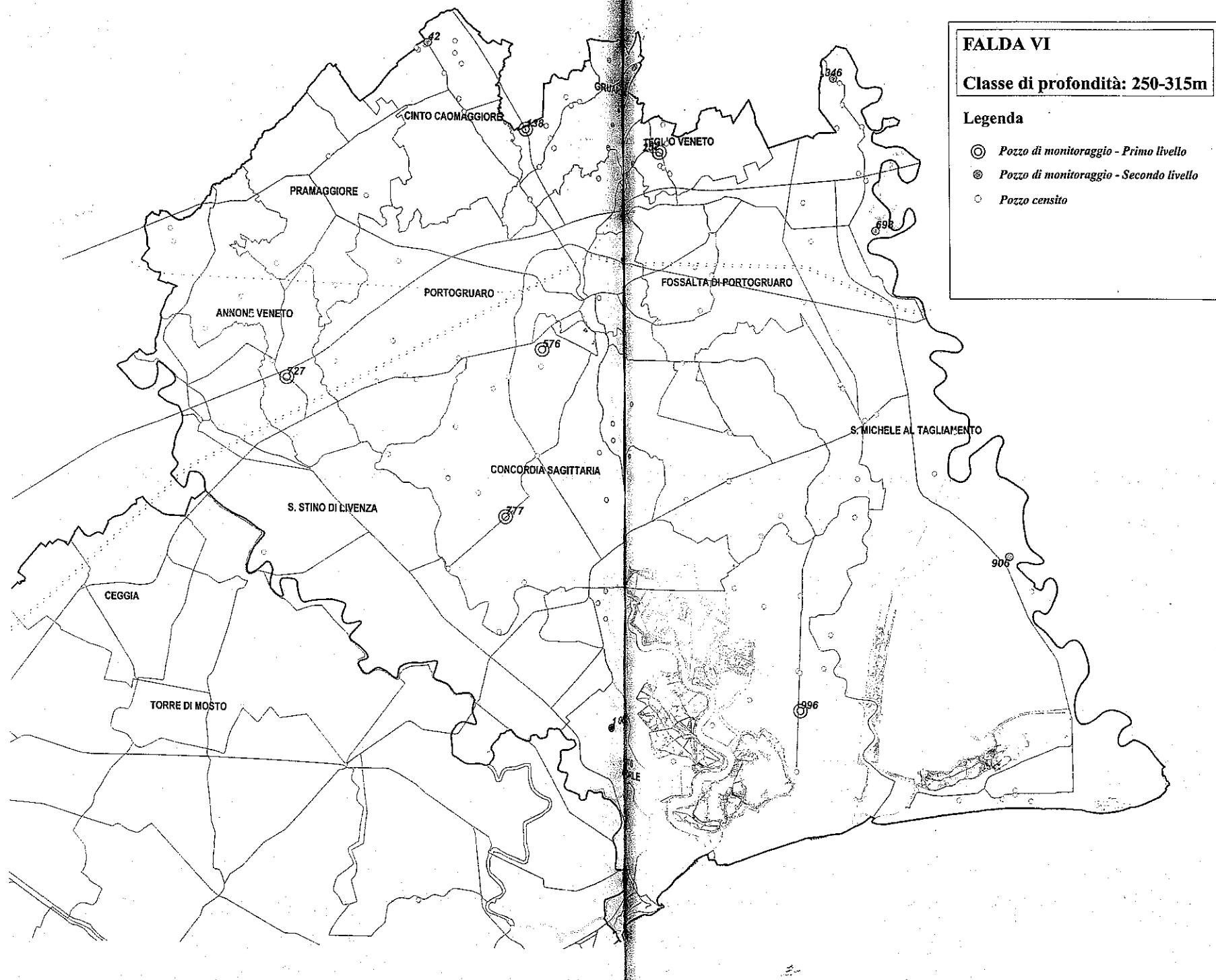
Figura 38 - Falda VI - Classe di profondità: 250-315. Pozzi censiti e rete di monitoraggio.
