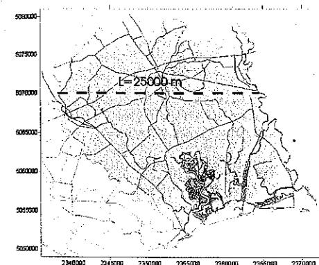
Figura 27 - Sezione Est-Ovest, posta all'altezza di Portogruaro per il calcolo delle portate delle falde.
