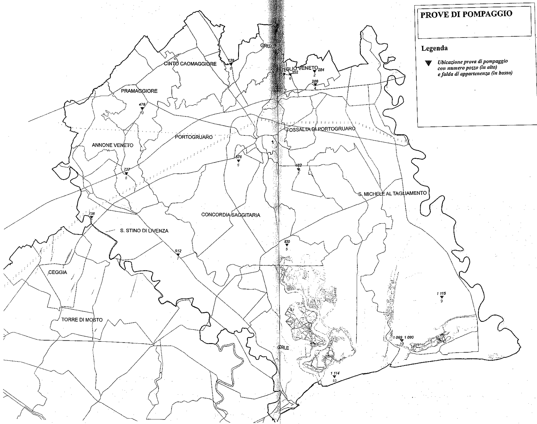
11 - Ubicazione dei punti su cui si sono realizzate le prove di pompaggio, con indicata la falda di appartenenza.
