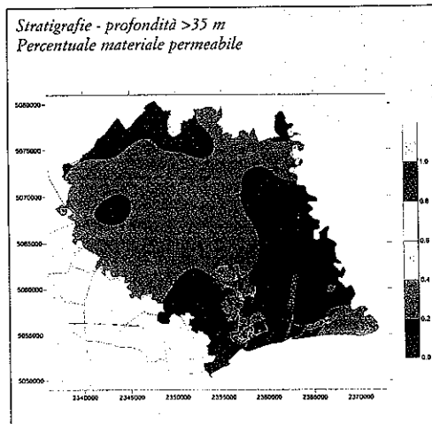
Figura 25 - Spessore dei materiali acquiferi (loro poroso: sabbia e ghiaia) espresso in percentuale, elaborato sulla base delle stratigrafie di profondità superiore ai 35 metri.
