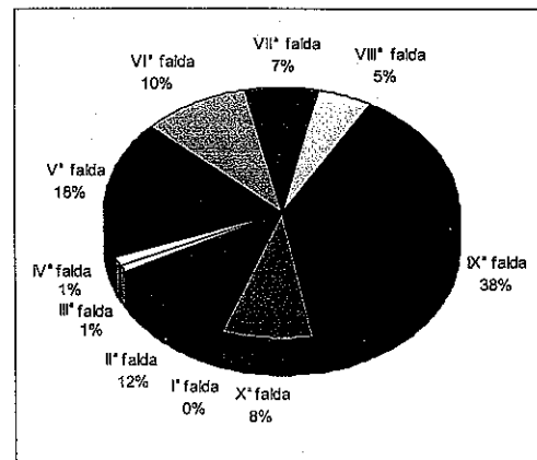
Figura 29 - Percentuale del consumo totale prelevato da ciascuna falda.
