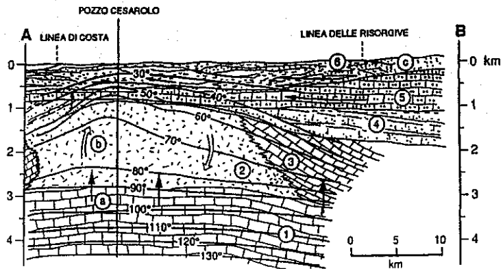
ura 22 - Schema del sottosuolo dell'area geotermica (da Bellani et alii) - 1) Dolomie e calcari dolomitici (Trias sup.-Lias); 2) care biogenico di piattaforma (Dogger-Cretaceo sup.); 3) Scarpa e calcare di bacino (Dogger-Cretaceo sup.); 4) Flysch (Paleocene); 5) Arenarie arcosiche (Miocene); 6) Depositi fluviali e marini (Quaternario); a) conduzione dominante; b) convenzione ninante; c) circolazione superficiale.
