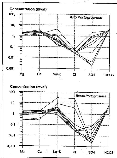
Figura 21 - Diagrammi di Schoeller (da Zangheri, 2000).
