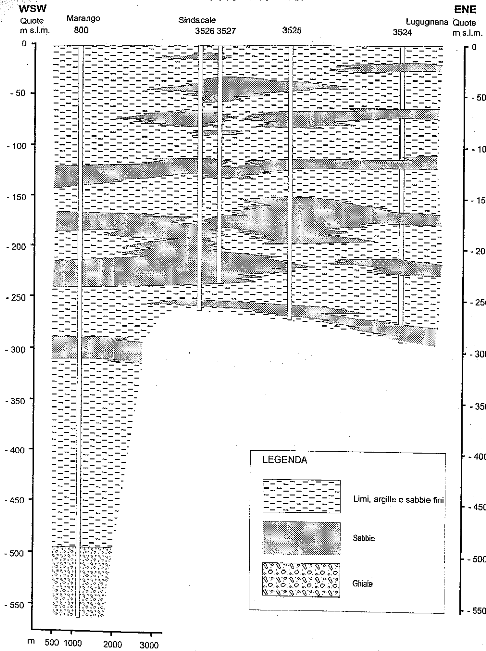
gura 5 - Profilo litostratigrafico N. 2.
