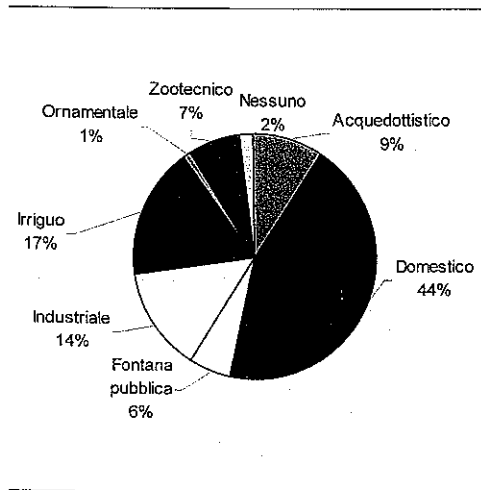
Figura 31 - Prelievi (percentuale sul totale) di acque sotterranee suddivisi per tipo di utilizzo.
