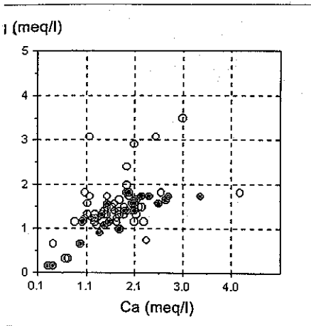
20 - Diagramma Calcio-Magnesio per l'intera provincia di Venezia; i pallini pieni corrispondono ai pozzi del Portogruarese.
