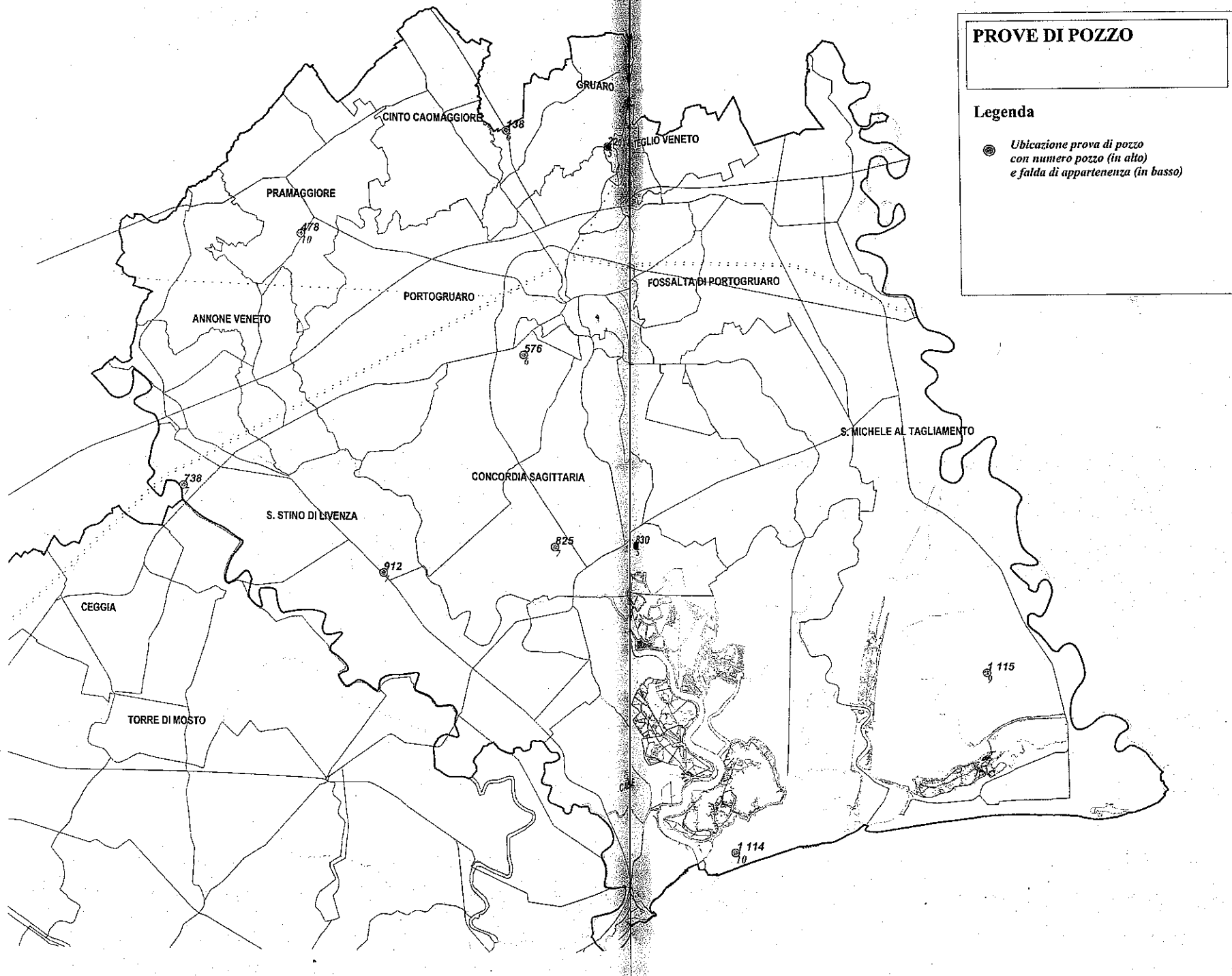
gura 10 - Ubicazione dei punti su cui si sono realizzate le prove di pozzo, con indicata la falda di appartenenza.
