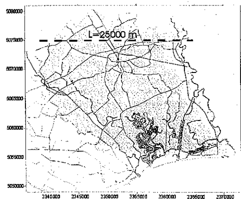
Figura 26 - Sezione Est-Ovest, posta in ingresso all'area di studio, utilizzata per il calcolo delle portate delle falde.
