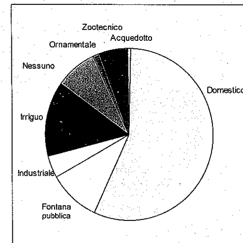
Figura 30 - Utilizzo prevalente dei pozzi (percentuale sul numero totale dei pozzi).
