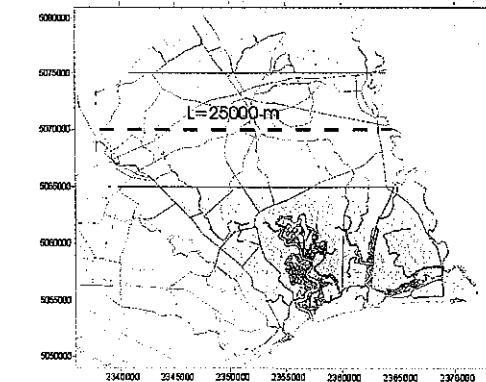
Figura 28 - Fascia sulla quale si è calcolato il gradiente idraulico medio.
